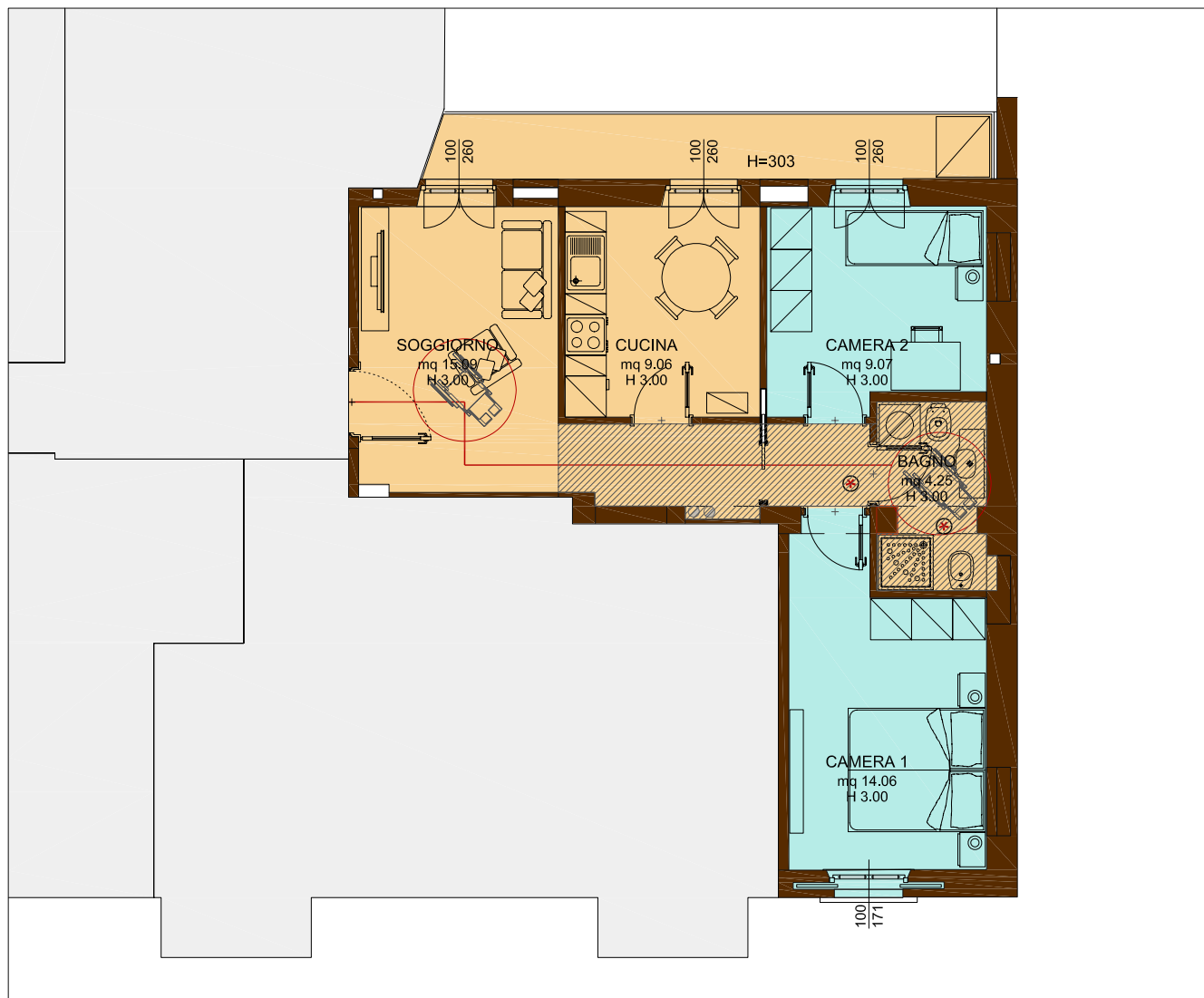
PIANTA UNITA' ABITATIVA A34 PIANO TERZO
